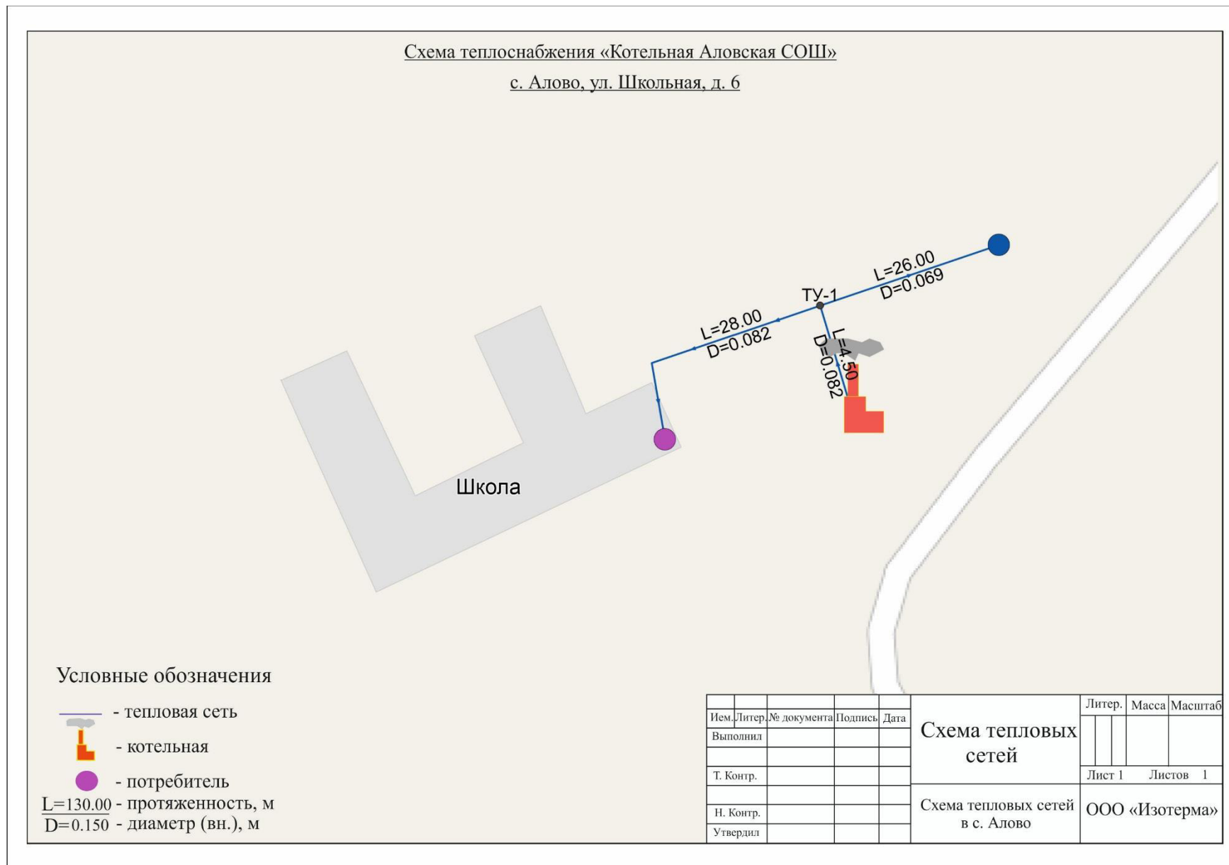
Рисунок 1. Зона действия котельной Аловская СОШ
